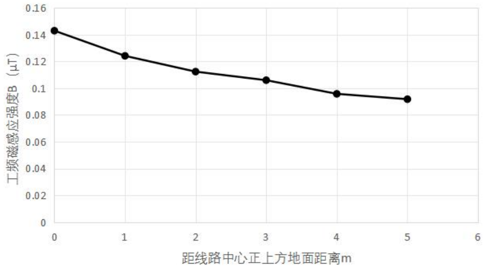
图 7-2 监测断面工频磁感应强度变化趋势图
