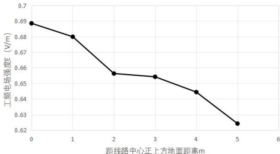
图 7-1 监测断面工频电场强度变化趋势图
